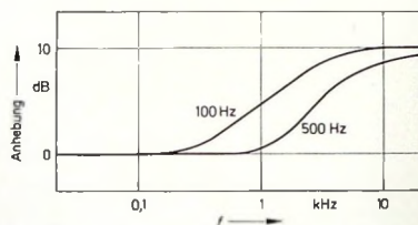
Bild 5. Automatische Verschiebung der Grenzfrequenz, oberhalb derer die Anhebung einsetzt. Dadurch wird die Gefahr der Übersteuerung durch Anhebung starker mittlerer Tonfrequenz-Komponenten vermieden
