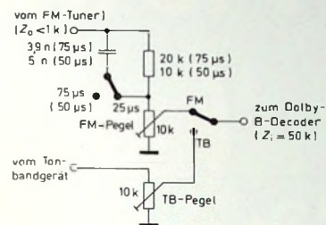
Bild 7. Schaltung für die wahlweise Verwendung eines Dolby-B-Decoders für die Wiedergabe dolbysierter FM-Rundfunksendungen oder Tonbandaufnahmen
