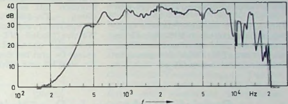
Bild 1. Mittelton-Hornlautsprecher „HM-450A“
