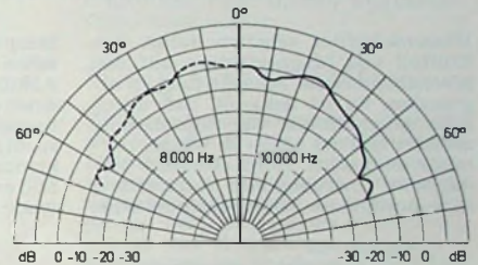
Bild 3. Polares Richtdiagramm des „HM-450A“ bei den Frequenzen 4000 Hz (unten links), 6000 Hz (unten rechts), 8000 Hz (oben links) und 10 000 Hz (oben rechts)
