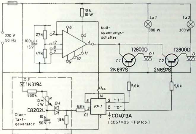
Bild 21. Schaltung einer Triac-Steuerung mit Nullspannungs-Synchronisation bei einer Blinkeinrichtung
