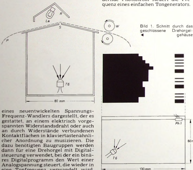
Bild 2. Schnitt durch das geschlossene Drehorgelgehäuse parallel zum Spalt
