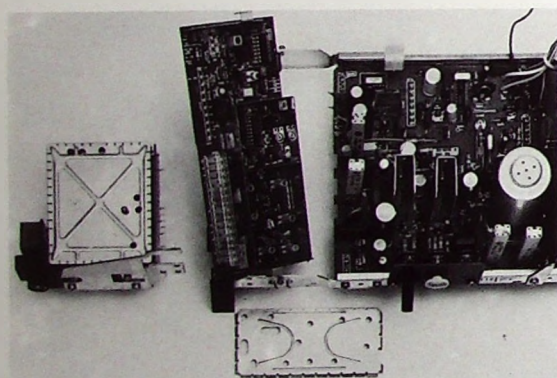
Bild 4 Tuner und Verstärker in ausgebautem Zustand
