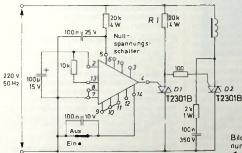
Bild 21. Schaltung einer Triac-Steuerung mit Nullspannungs-Synchronisation bei einer Blinkeinrichtung
