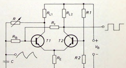
Bild 3 (unten). Prinzipschaltung des Licht-Frequenz-Wandlers
