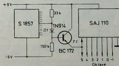
Bild 3. Anschluß von Oktavteilern SAJ 110 an den MOS-Baustein S 1857
