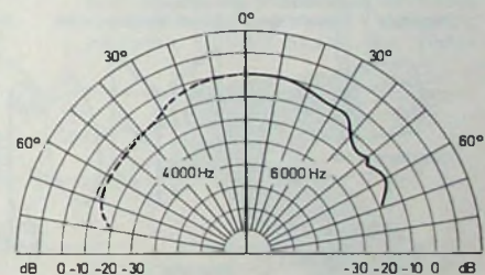
Bild 5. Super-Hochton-Lautsprechersystem „TW-3300A“
