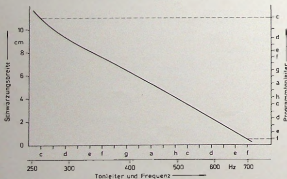
Bild 8. Programmstreifen zur Aufnahme der Eichkurve
