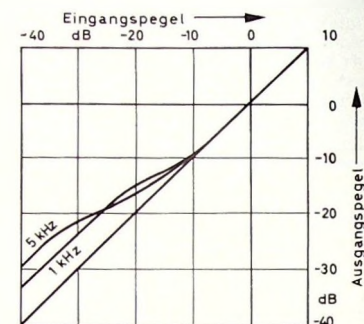
Bild 4. Übertragungskennlinien eines Dolby-B-Coders. Die bevorzugte Anhebung der höheren Frequenzen bei niedrigen Pegeln ist deutlich erkennbar
